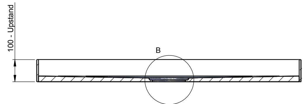
SECTION A-A SCALE 1 : 10
